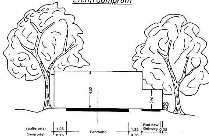
Lichtraumprofil
